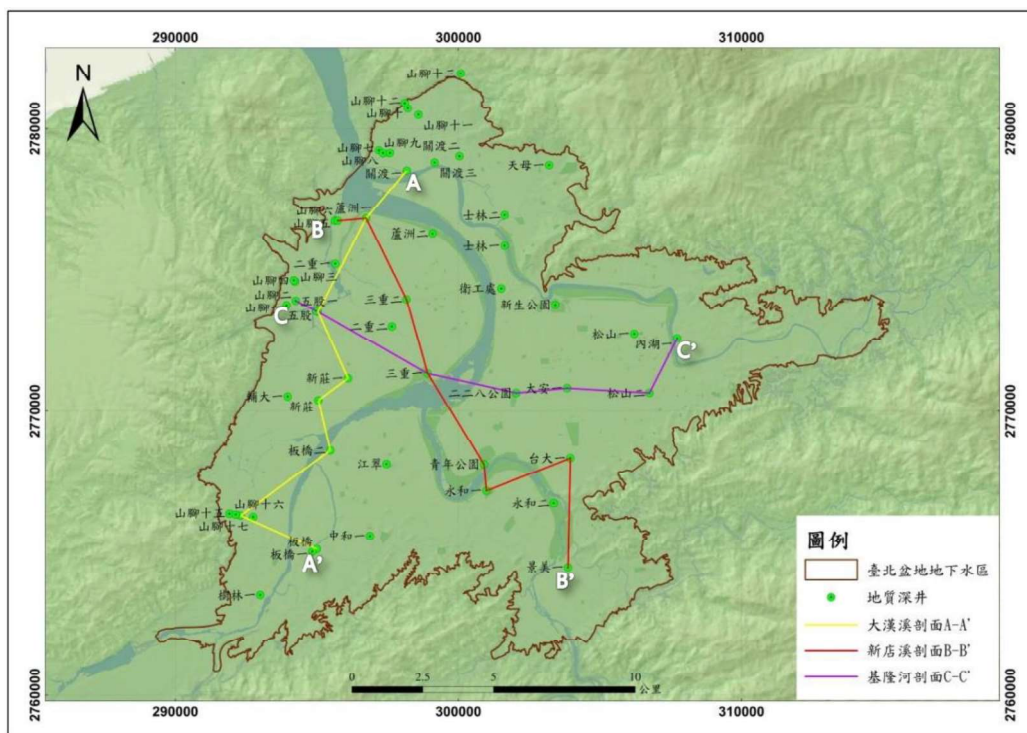
圖 1 臺北盆地水文地質剖面分布圖
