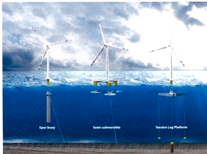
圖 4-4 浮體平台技術型式示意圖
