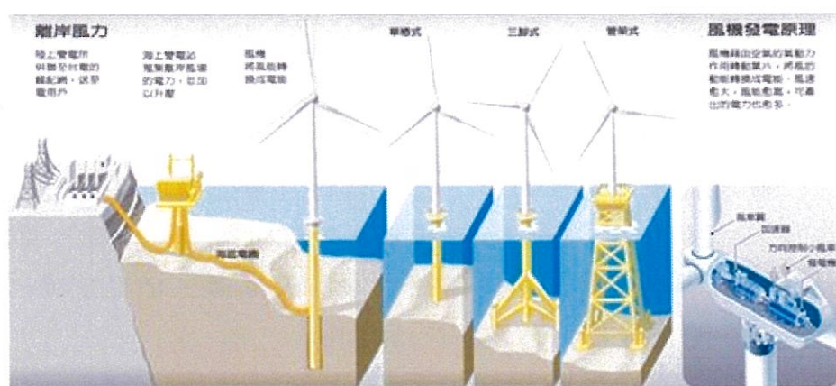
圖 4-11 固定式離岸風機基座與發電示意圖
