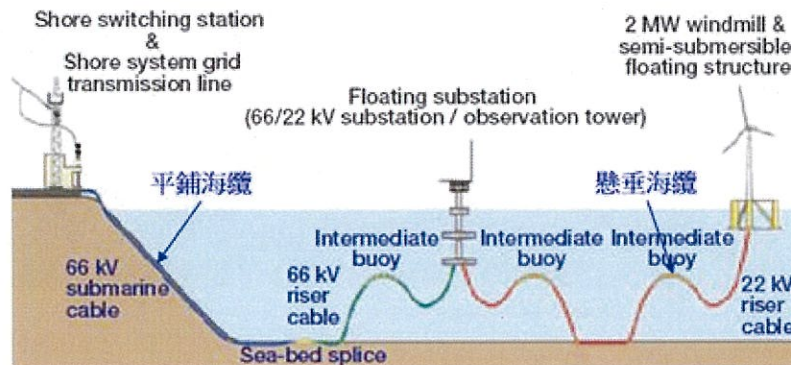
圖 4-5 浮動式離岸風機之海纜型態示意圖
