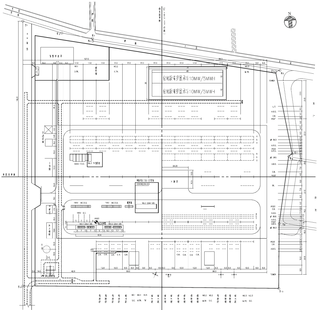
圖 22 路園 D/S 平面配置示意圖
