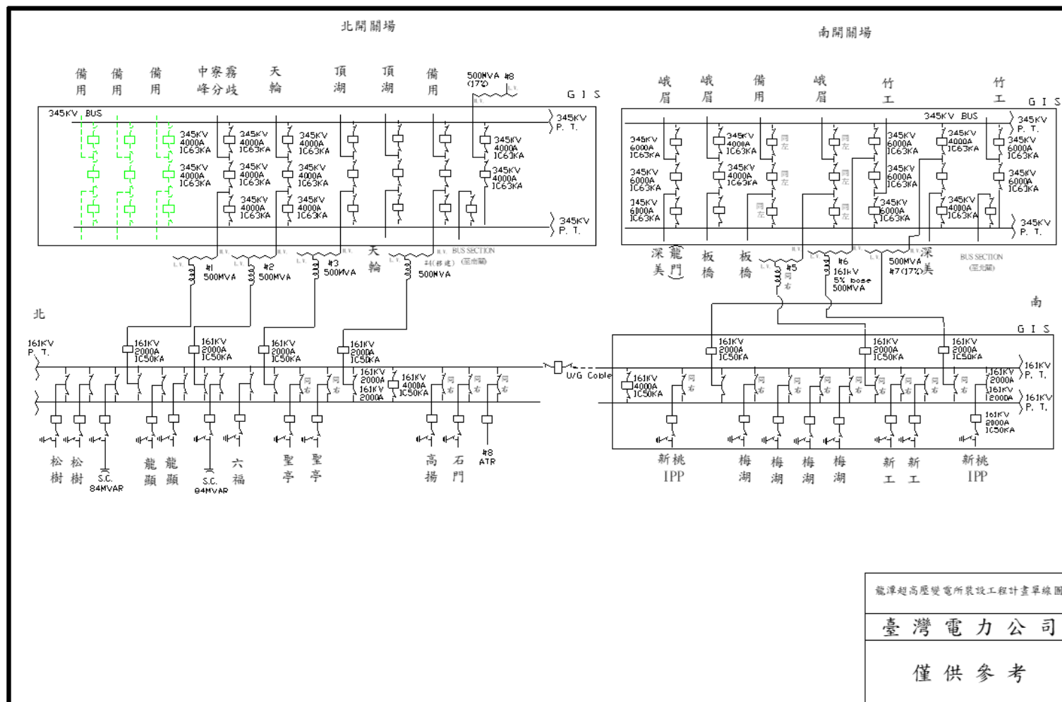
圖 28 龍潭 E/S 單線示意圖
