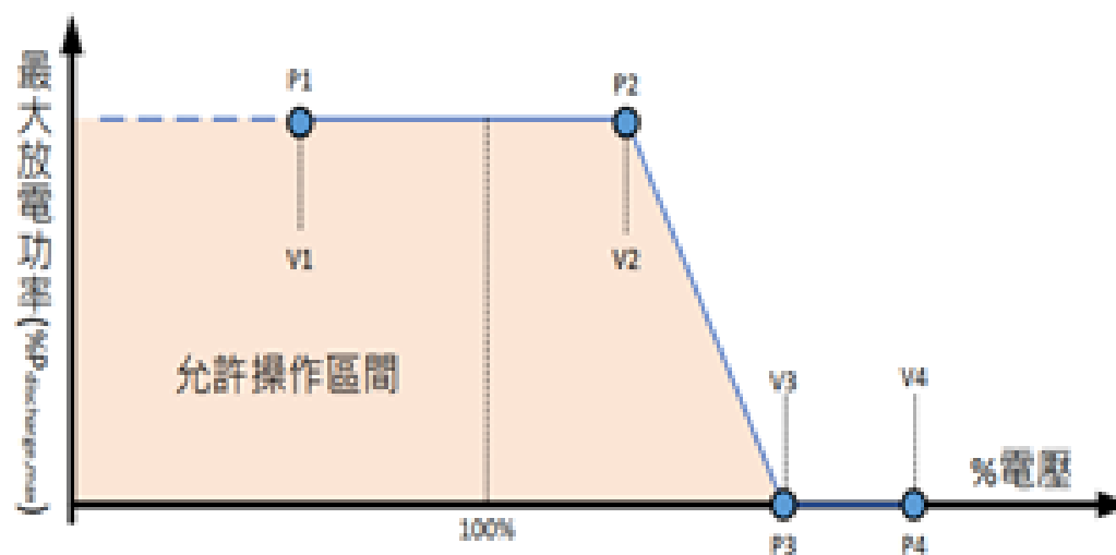
圖 37 Volt-Watt 操作點示意圖
