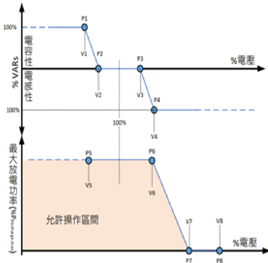
圖 38 Volt-Var 與 Volt-Watt 同時操作示意圖
