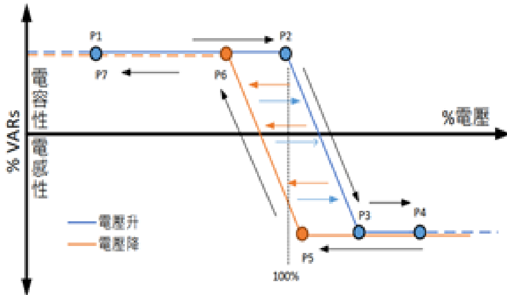
圖 36 Volt-Var 操作點示意圖
