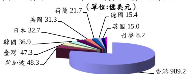
圖3-2 前十大外資國/地區 2017年1-12月實際投資金額（非金融領域）比重95.1%
