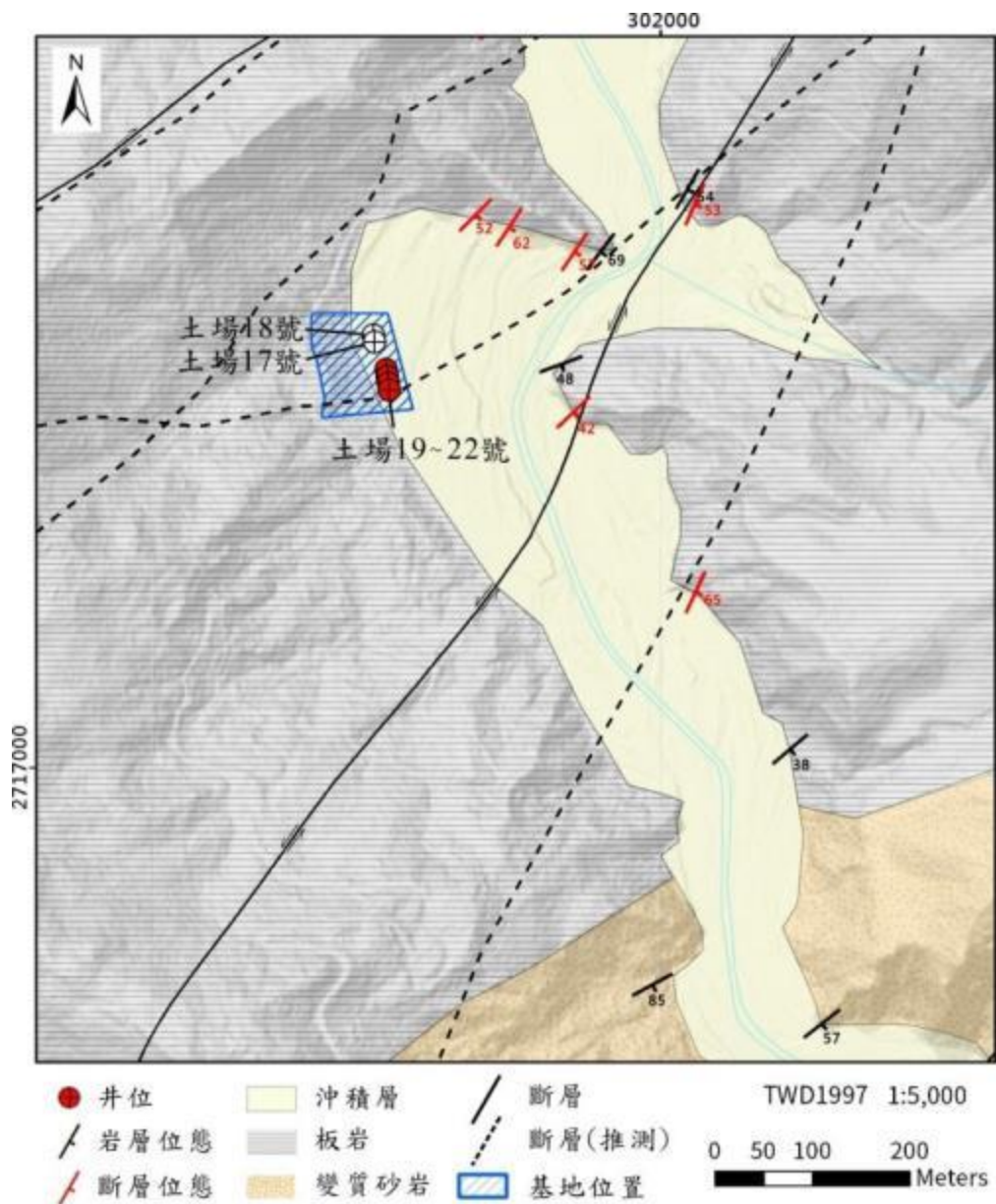
圖4-7 基地地質圖。
